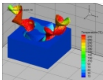
IDCH shown less cutting heat IDCH가 절삭열이 작게 발생함을 보여줌
