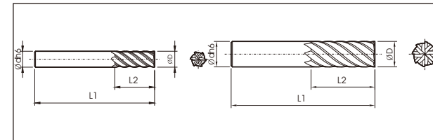
YSET/HH
