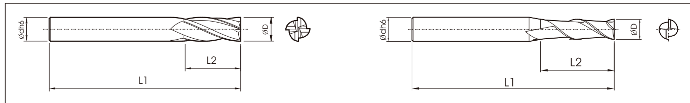
YSET-4F
