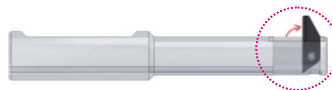
Blade is exposed by centrifugal force 회전시 원심력에 의해 날이 펴짐
