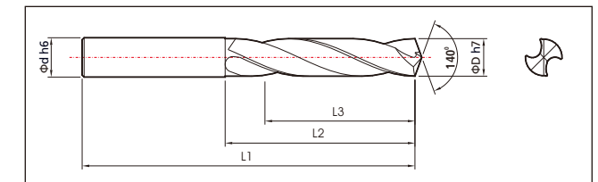
YSDL TiAlN
